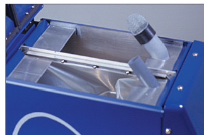
Großer Tank mit Trennmembran für Frisch- und Schmutzwasser (Flextank)
